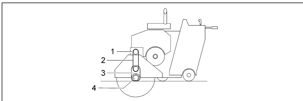
Entraînement de la lame de scie (schéma)
